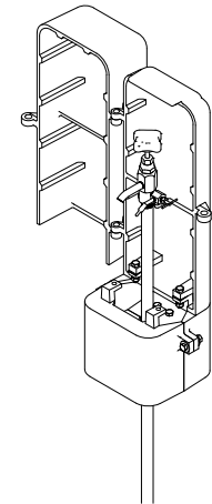
C ISO VIEW Scale: 3/4"=1'-0"
