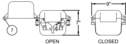
B TOP VIEWS Scale: 3/4"=1'-0"
